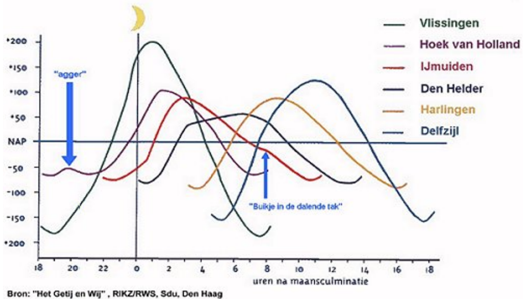
Afb. 3 Getijcurves langs de Nederlandse kust ( Uit: Het Getij & Wij , Rijkswaterstaat , RIKZ, Sdu, Den Haag, 1996. In deze afbeelding hierboven vinden we de getijkrommen van Vlissingen tot en met Delfzijl, in amplitude en tijdsduur. Qua vorm zijn ze allemaal verschillend. Op sommige plekken, zoals bij Hoek van Holland, ook nog een beetje bij IJmuiden, zit een merkwaardig klein bultje in de dalende tak. M.a.w.: nadat het water grotendeels is gevallen vindt eerst nog een kleine rijzing plaats, waarna het definitief valt tot het laag water zal zijn. Wanneer zo'n bultje echt duidelijk waarneembaar is noemt men dat een 'aggr'
