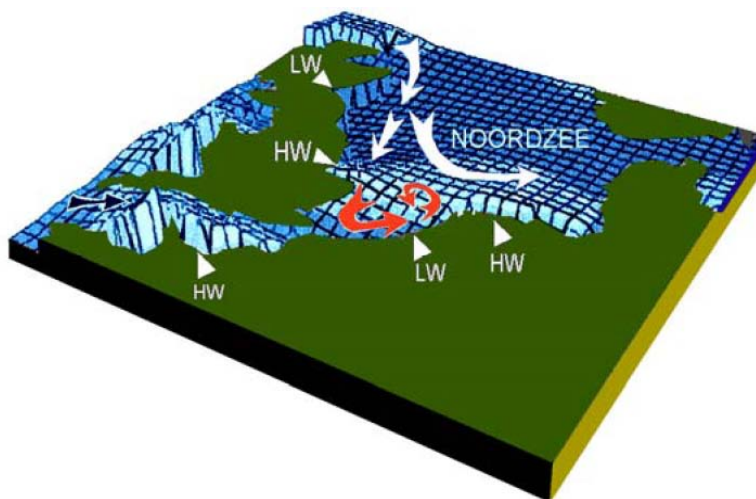
Afbeelding 1. De oorsprong van het getij ligt op het zuidelijk halfrond. Vandaar plant het zich over de oceanen in noordelijke richting voort. Zo ook over de Atlantische Oceaan. Ten noorden van Schotland buigt het de Noordzee binnen en loopt het langs de Britse kust zuidwaarts tot een stuk voor het Nauw van Calais alvorens weer in een noordoostelijke richting langs de Belgische, Zeeuwse en Hollandse kusten te gaan lopen. Ter hoogte van de Wadden buigen ze tenslotte af naar het midden van de Noordzee
